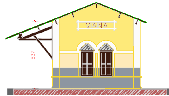
Fachada Fundos ESC.: 1/50
