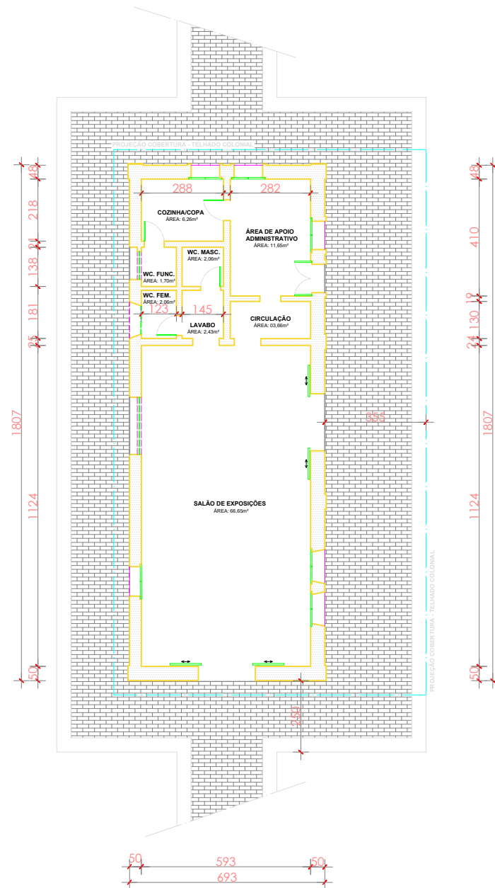
Planta Baixa ESC.: 1/50
