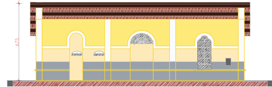
Fachada Esquerda ESC.: 1/50
