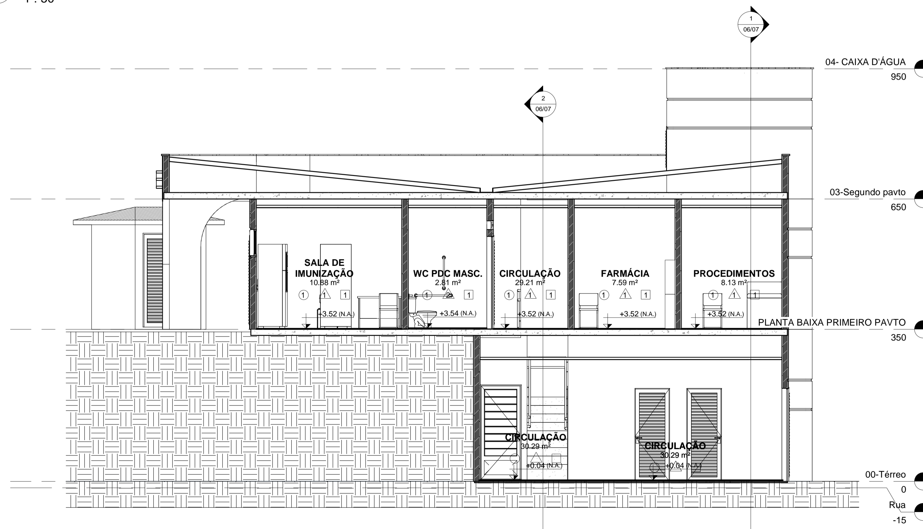
2 CORTE 02 F6 1:50
