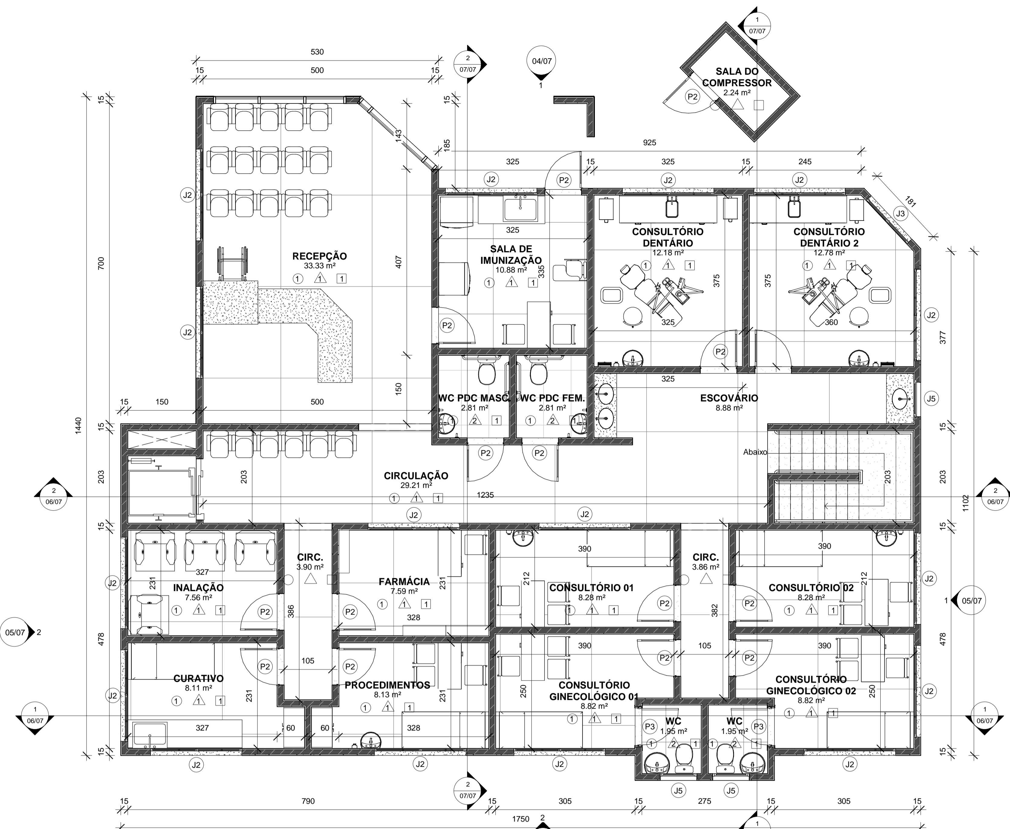
1 PLANTA BAIXA PRIMEIRO PAVTO 1 : 50
