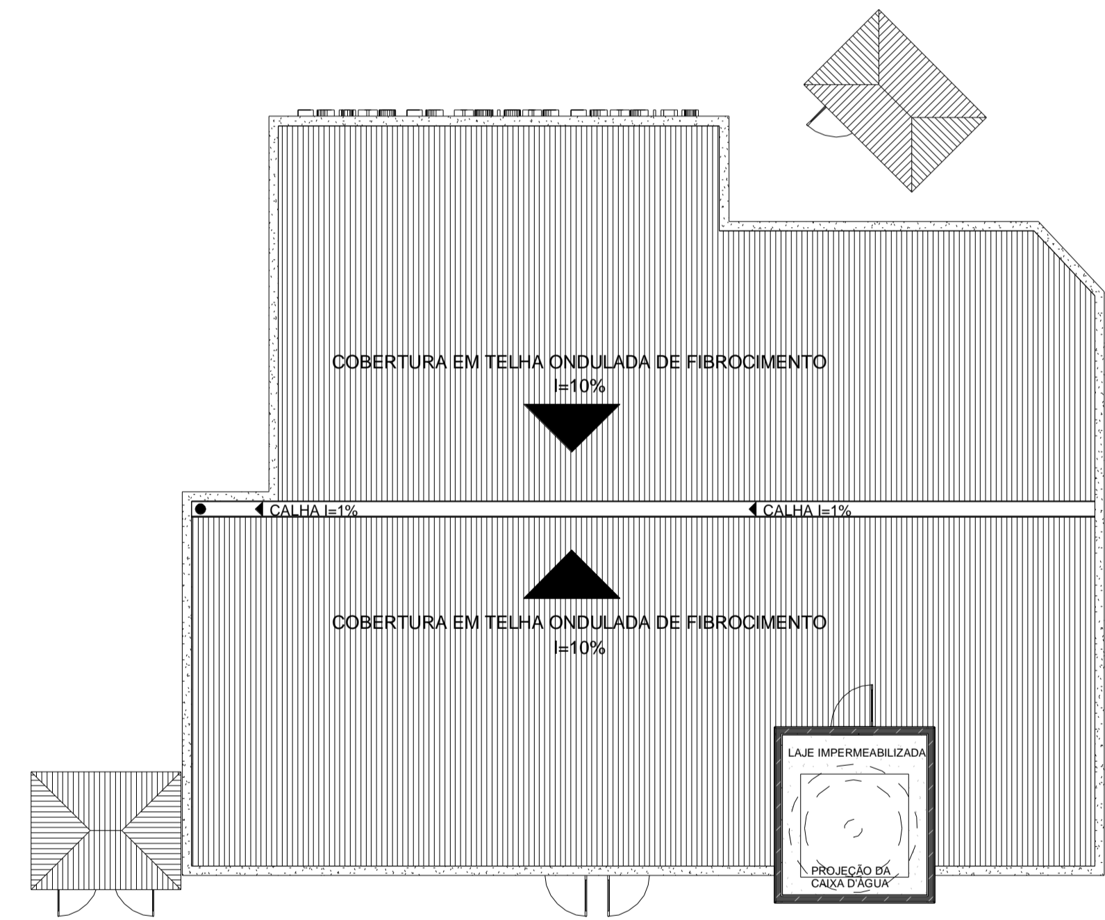
3 Planta de Telhado 1 : 100
