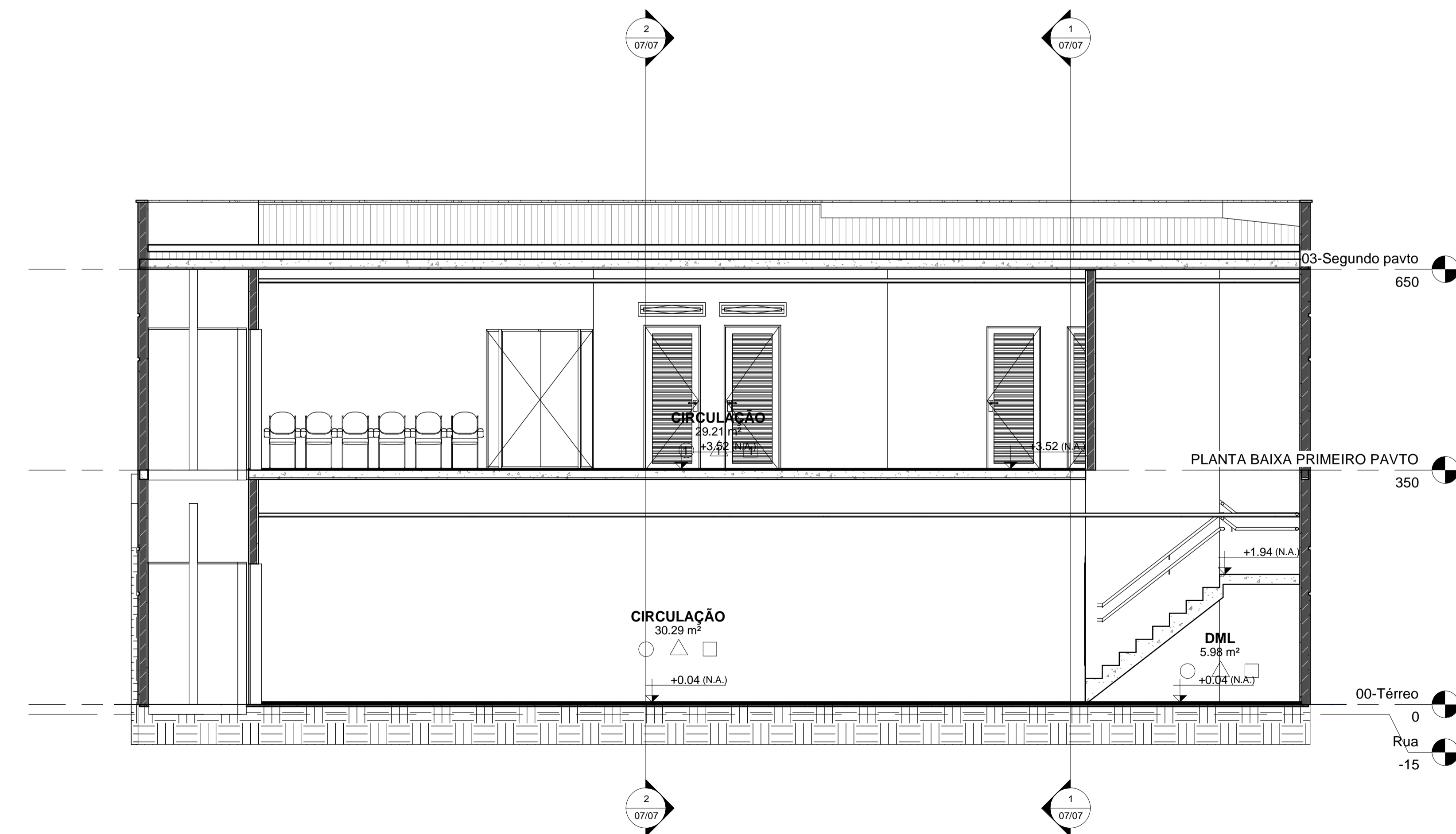
2 CORTE 02 F5 1:50
