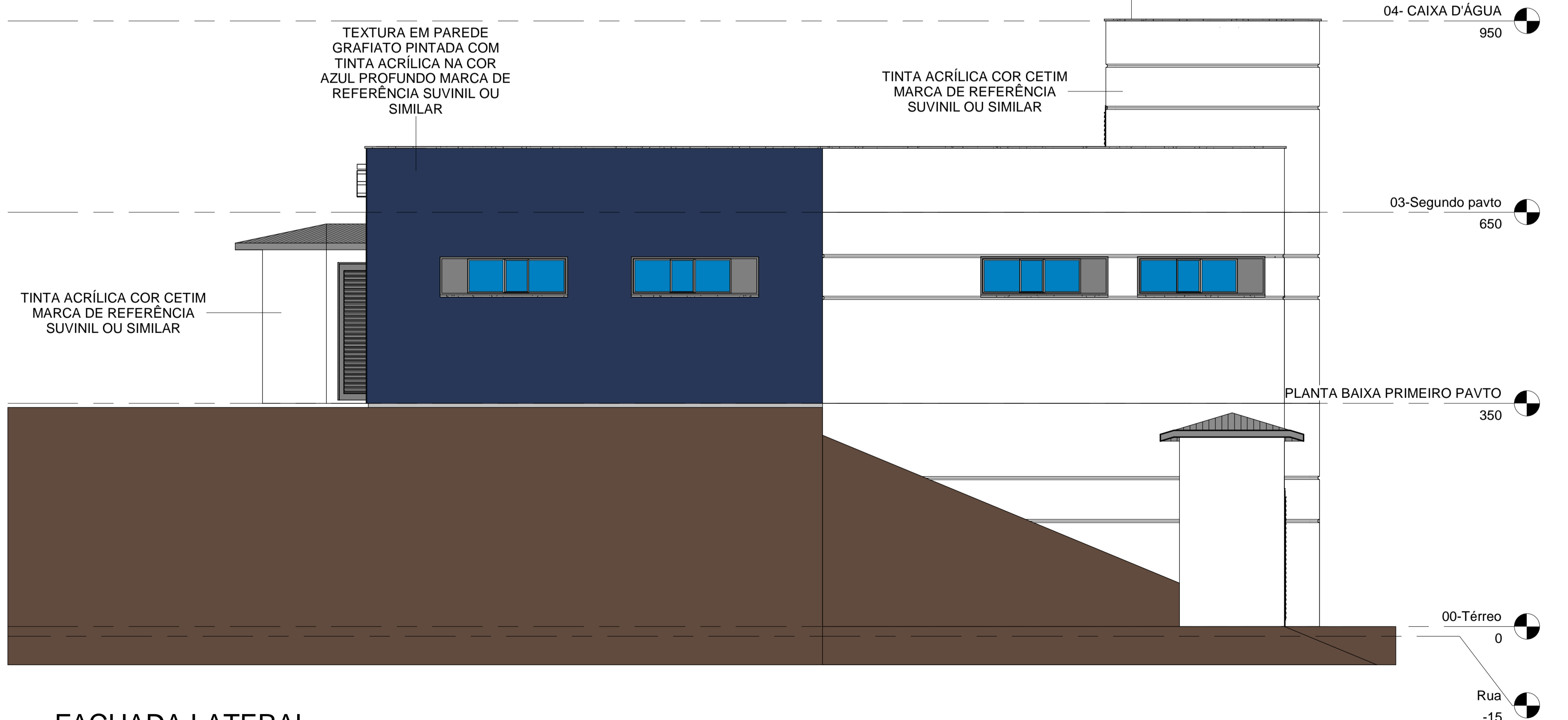
2 FACHADA LATERAL DIREITA 1:50
