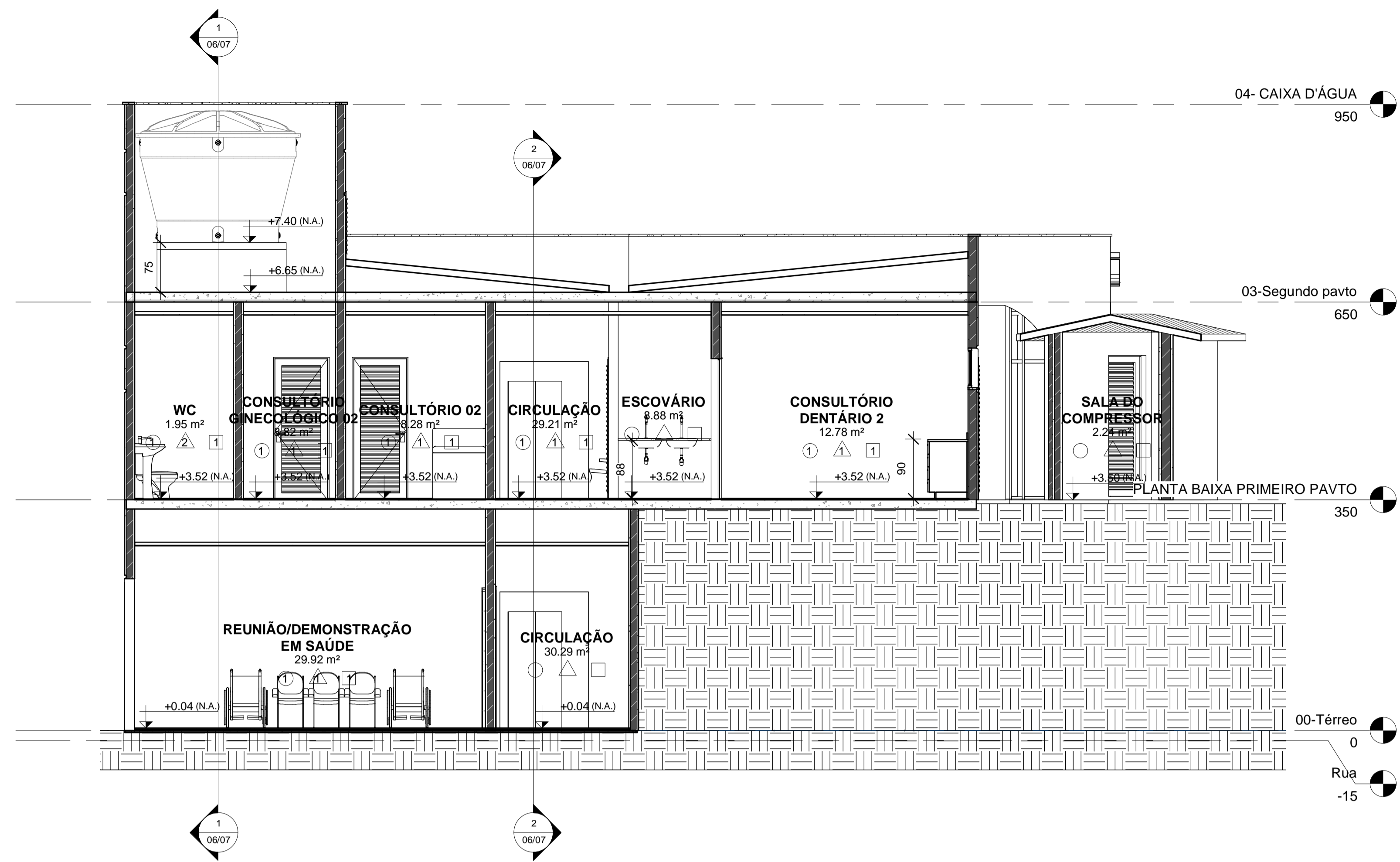
1 CORTE 01 F6 1:50
