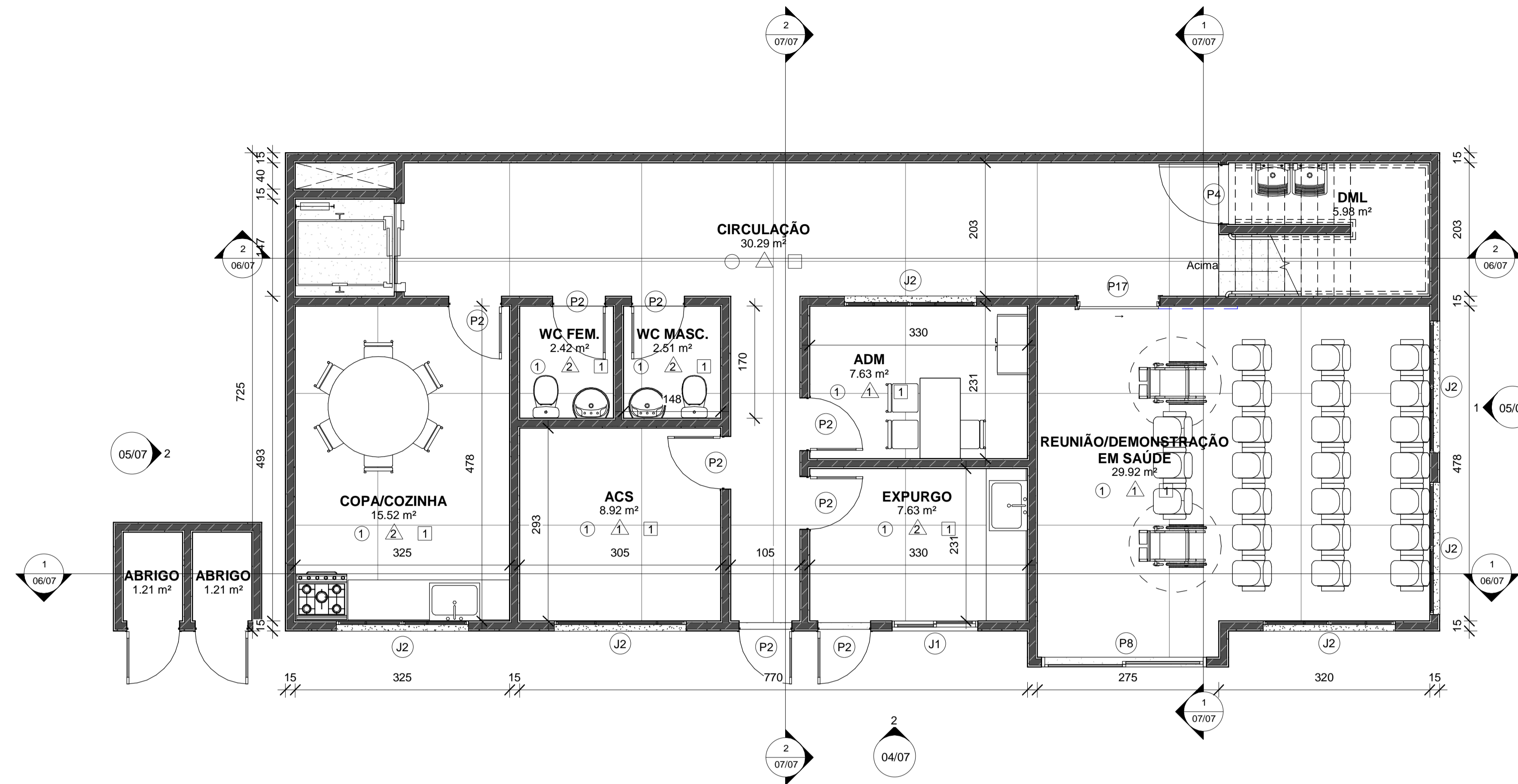
1 PLANTA BAIXA TÉRREO 1 : 50
