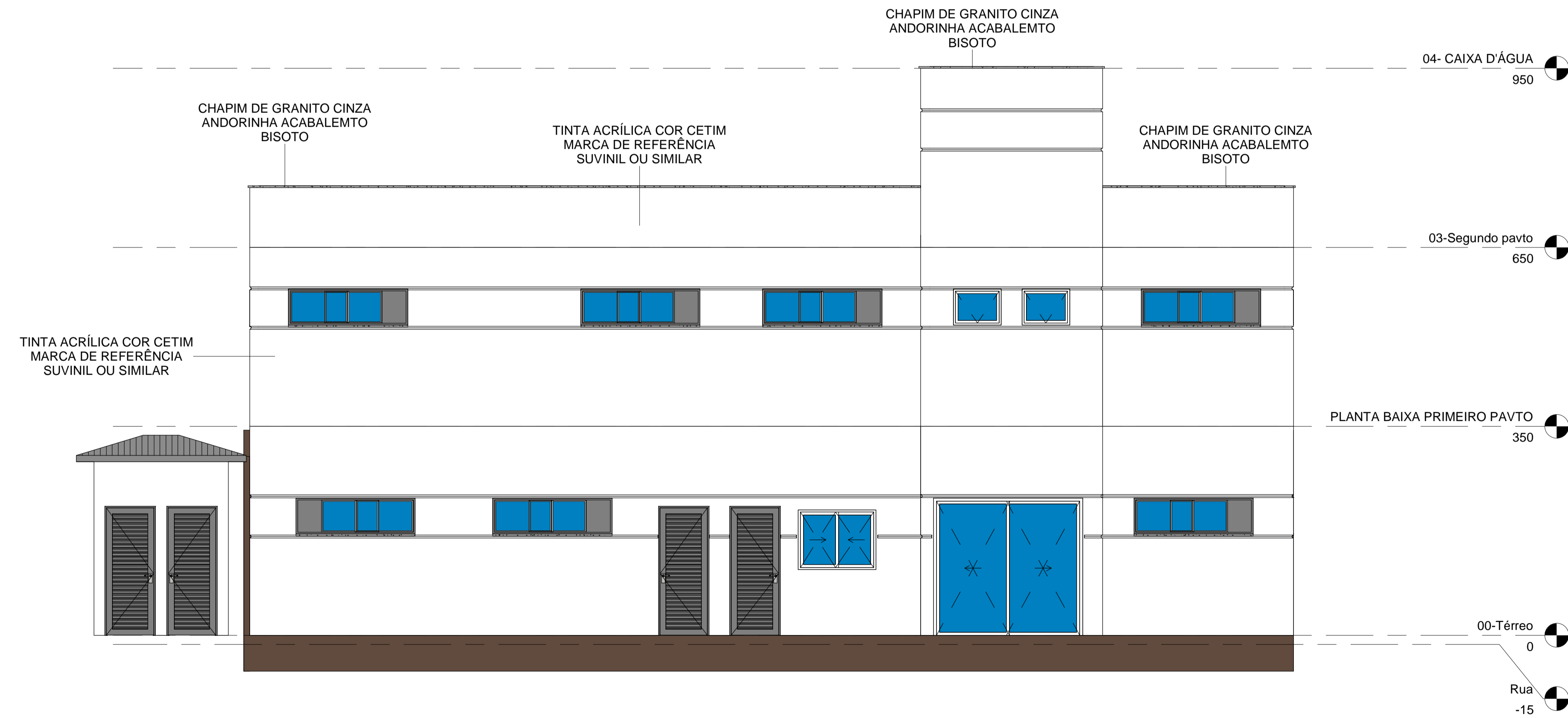
2 FACHADA FUNDOS 1 : 50
