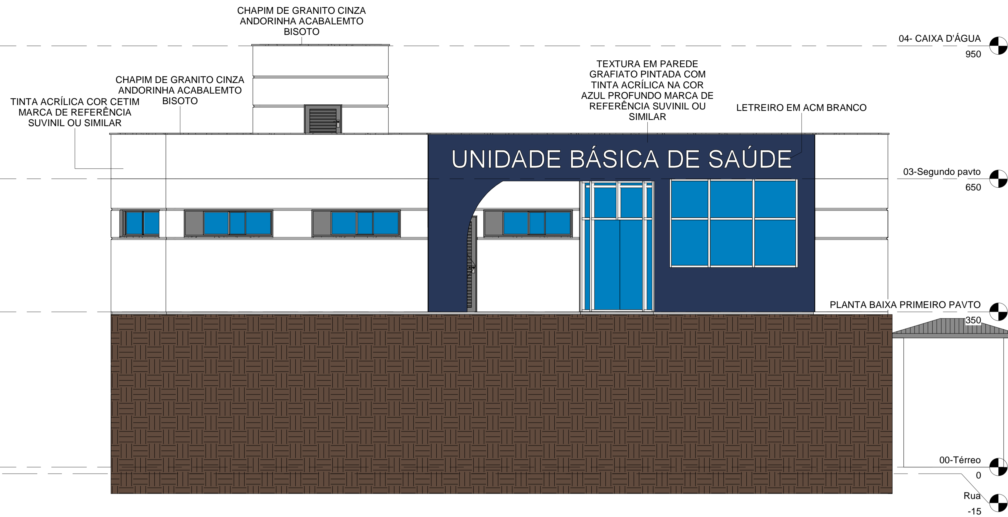
1 FACHADA FRONTAL 1 : 50
