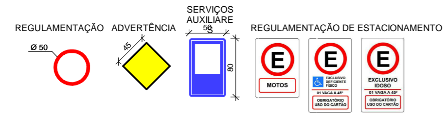
2 DET. SINALIZAÇÃO VERTICAL 1 : 50
