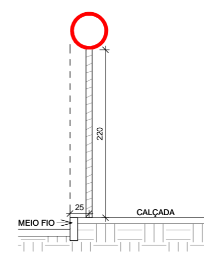
3 DET. PLACA 1 : 50
