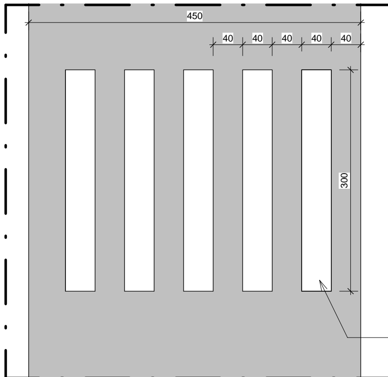
1 DET. FAIXA DE PEDESTRE NIVELADA 1 : 50
